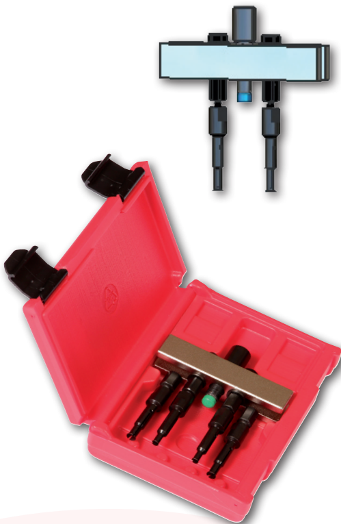
Inyector bomba Volkswagen Volkswagen pump injector
